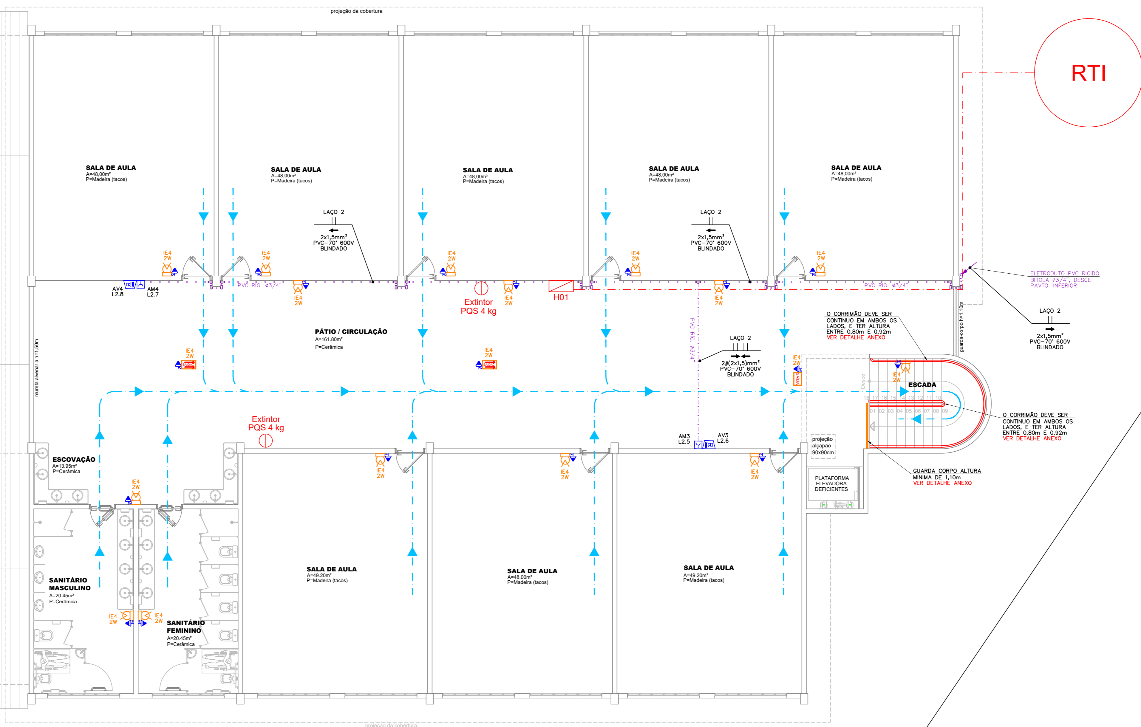
Planta Baixa 1º Pavimento Escala 1:75
