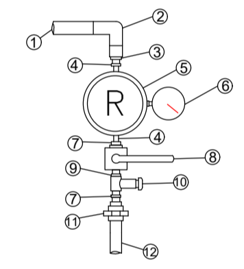
DET. DA CAIXA DE MANOBRA SEM ESCALA
