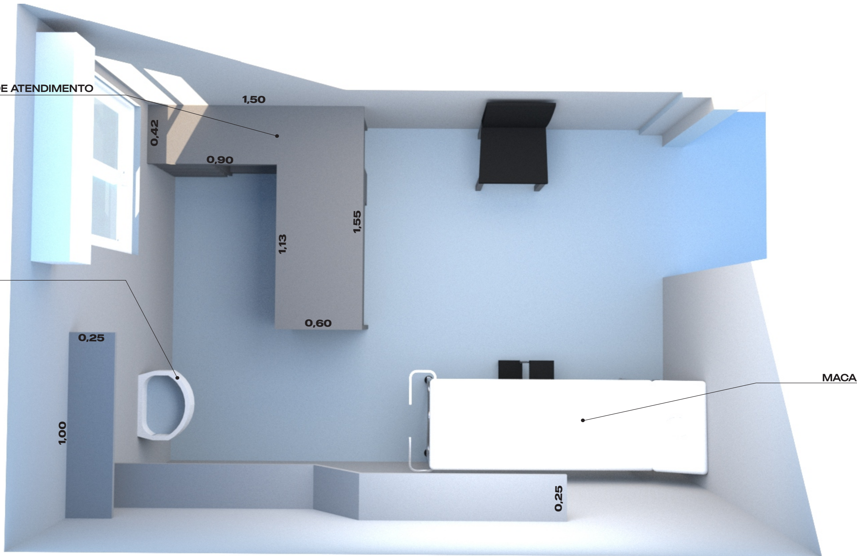
PLANTA BAIXA GERAL
