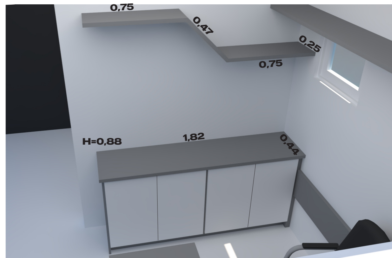
VISTA BALCÃO AUXILIAR LATERAL
